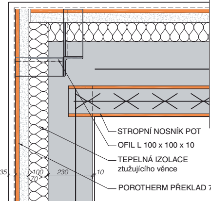
ŘEZ 2-2 PŮDORYSNÝ ŘEZ V ÚROVNI STROPU POROTHERM
