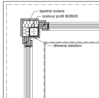
ŘEZ 2-2 PŮDORYSNÝ ŘEZ V ÚROVNI STROPU POROTHERM
